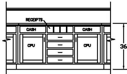
12 ELEVATION
